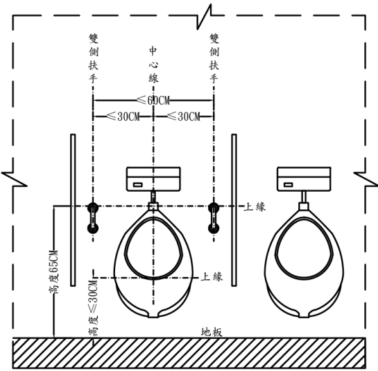
圖3-2（扶手上緣距地板面距離）
