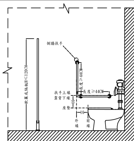
圖2-2(側邊 L 型扶手)
