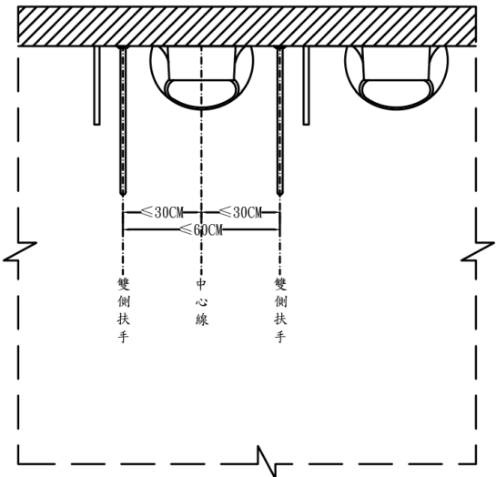
圖3-1（雙側扶手距離）
