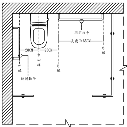
圖2-3 (扶手外緣與大便器中心線距離)
