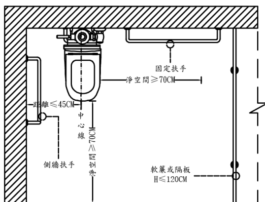
圖2-1(側邊淨空間)
